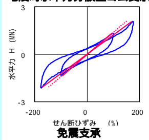
履歴曲線の例
