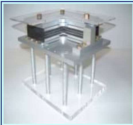
鉛プラグ入り積層ゴム支承
