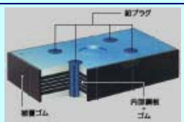
鉛プラグ入り積層ゴム支承
