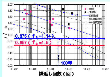
疲労耐久性試験結果
