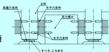
弾性支持型の例
