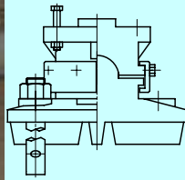
球面支承
