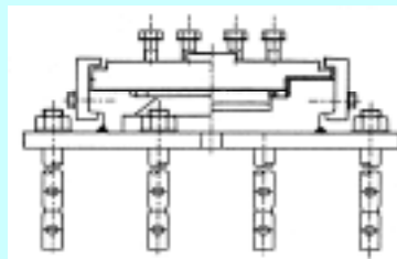
機能一体型の支承 (支承板支承)
