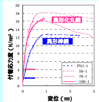
引抜試験結果
