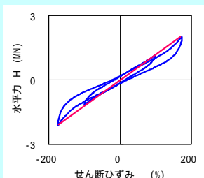
地震時水平力分散型ゴム支承
