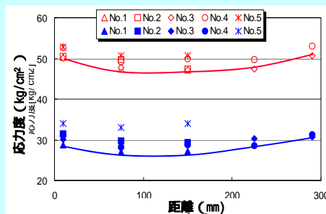
肉厚300mmの質量効果の例
