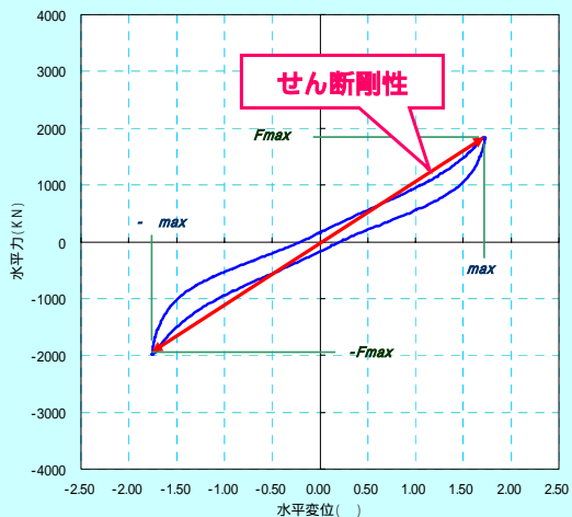
せん断剛性の模式図
