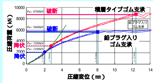
圧縮限界試験結果
