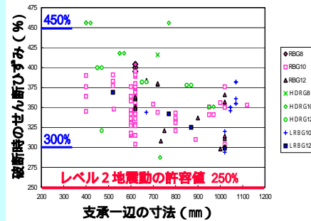
せん断変形性能試験結果
