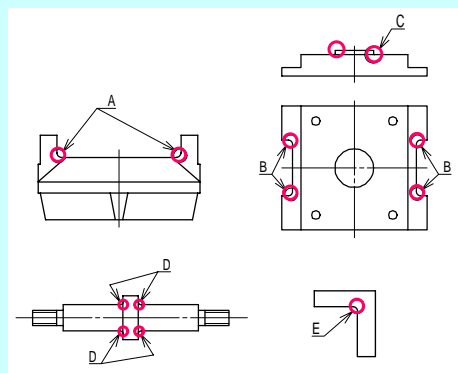
応力集中緩和する箇所
