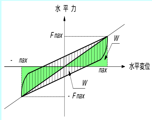
等価減衰定数の模式図
