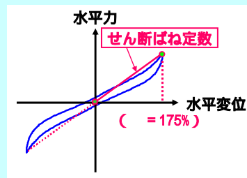
水平力 - 水平変位関係
