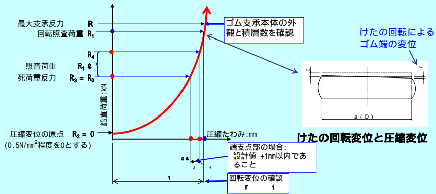
鉛直荷重 鉛直変位の関係
