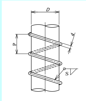
異形化丸鋼
