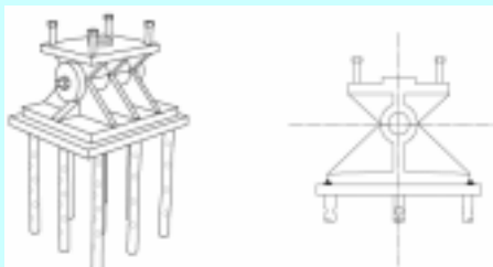
円柱面支承
